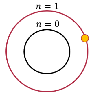
stato eccitato
