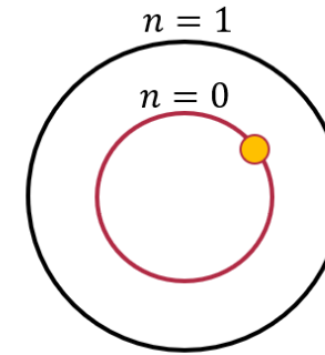
stato base
